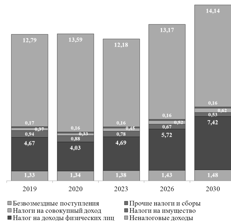
Рис. 8.3 – Прогноз основных характеристик бюджета города Ярославля, млрд руб.
