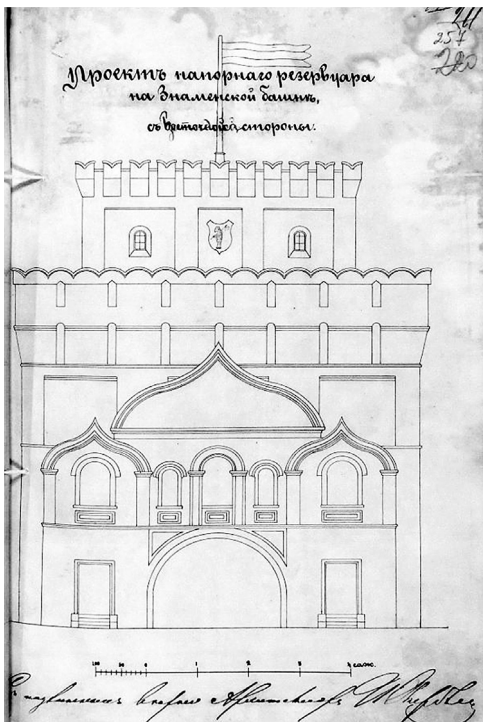
↓ Проект устройства напорного резервуара городского водопровода в Знаменской башне города Ярославля, разработанный в 1882 году.
